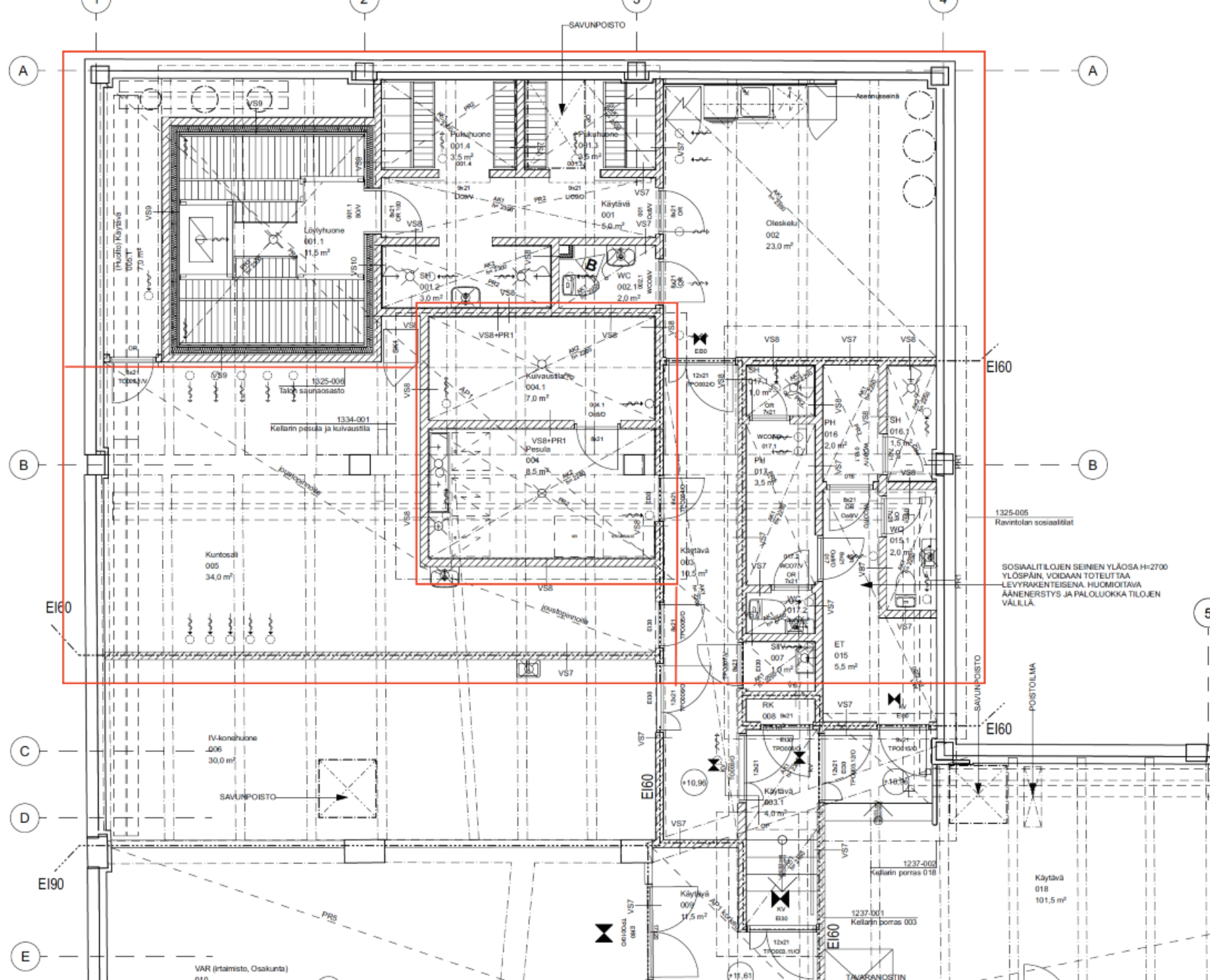
Kellarin uuden saunaosaston pohjapiirros
